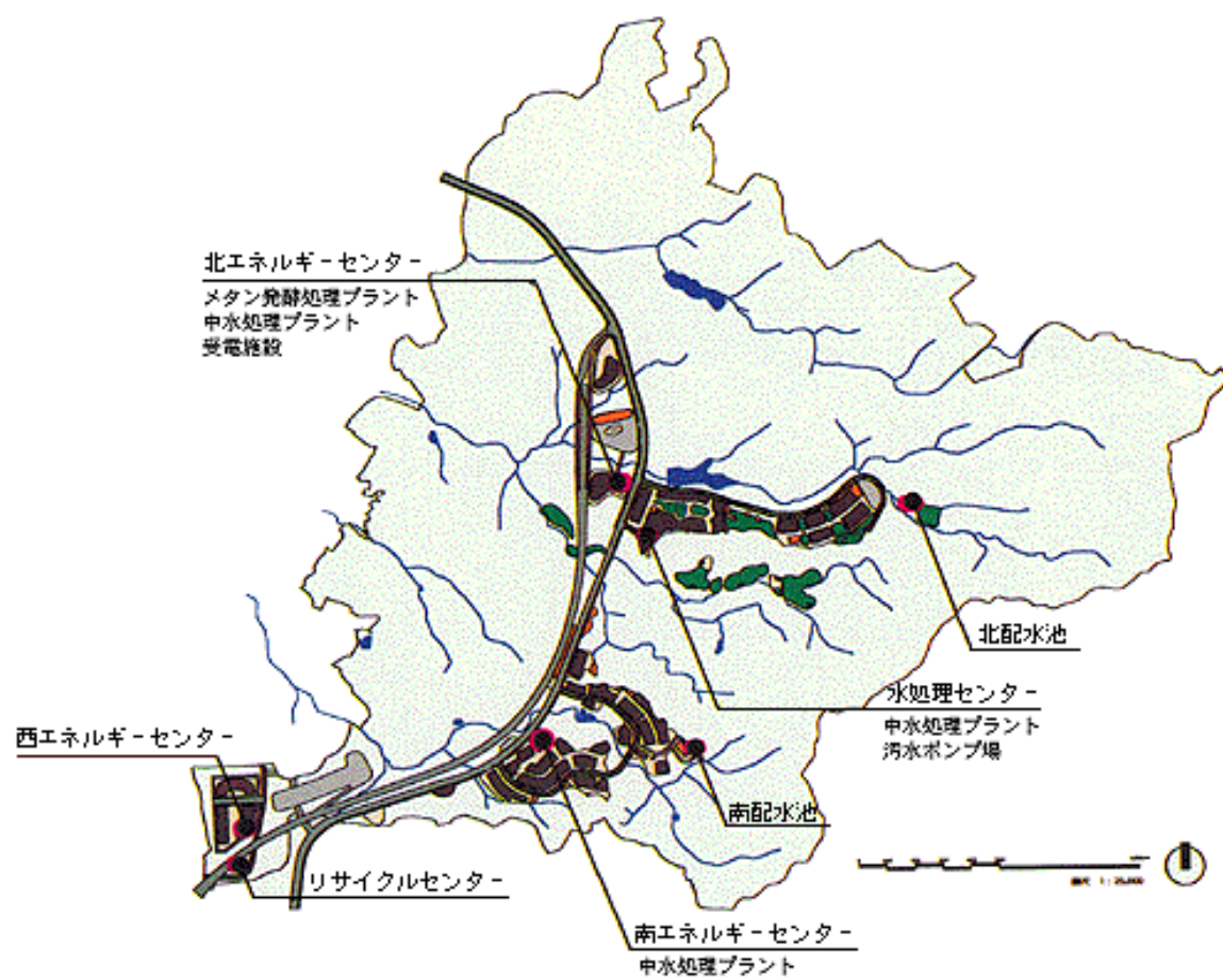
図 2 - 2 - 3 供給処理施設配置図
